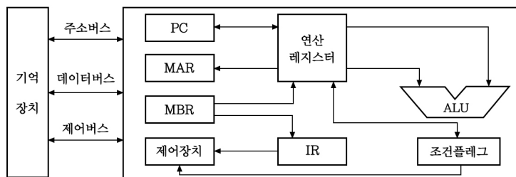
[중앙처리장치의 구성요소]
